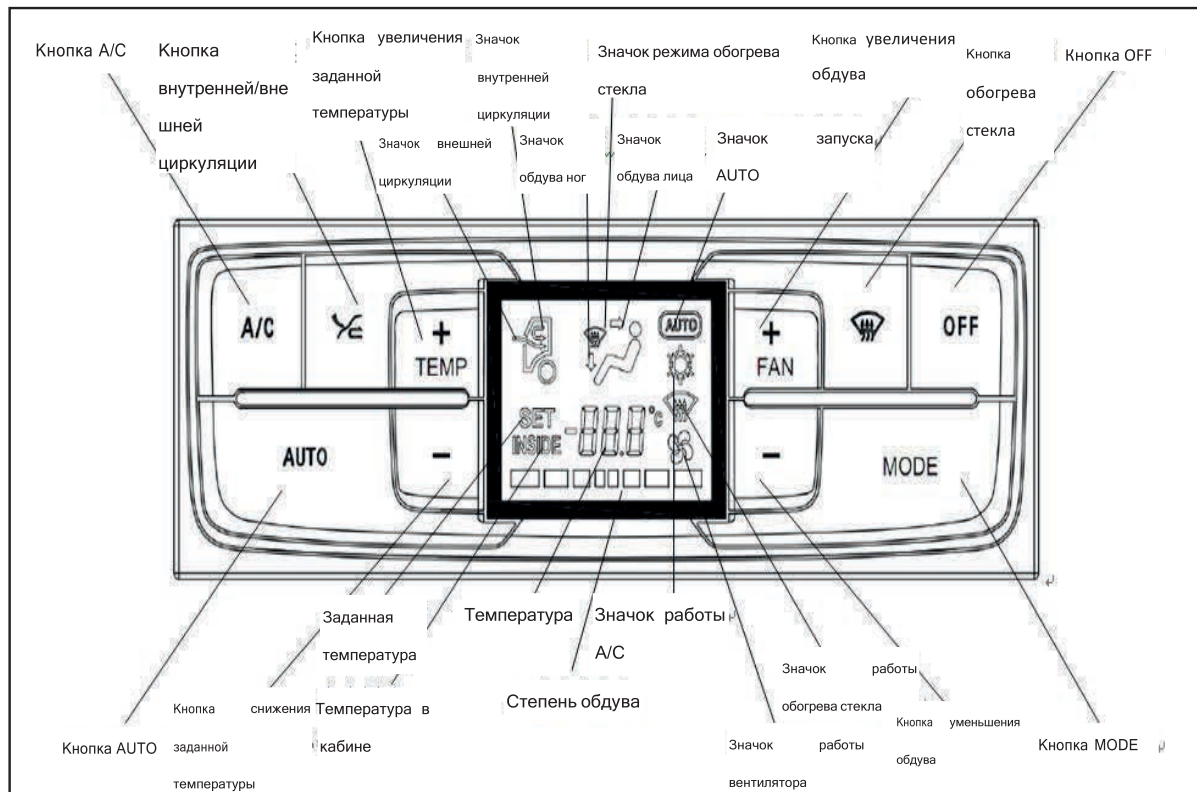
Устройство панели управления
